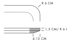
ECKE GERUNDET, KANTE AGESCHRÄGT/ ROUNDED CONER, BEVELLED EDGE
