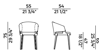
942/PAE poltrona pozzetto \ tub chair
