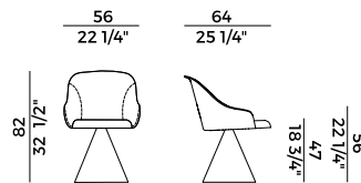
918/GCI sedia girevole \ swivel chair
