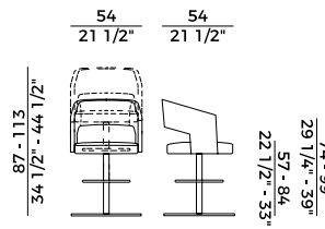
751/AII-GAS sgabello \ stool
