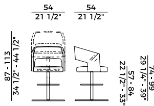
751/AI-GAS sgabello \ stool
