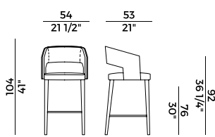
751/AIIW sgabello alto \ barstool
