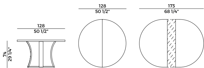
834/TC1 tavolo estensibile \ extendable table
