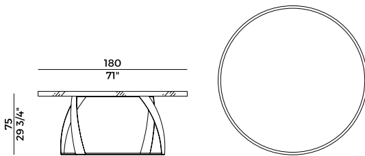
770/TG-C tavolo \ table
