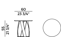
770/TB tavolino \ coffee table
