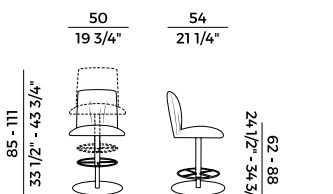
840/A-GAS sgabello \ stool
