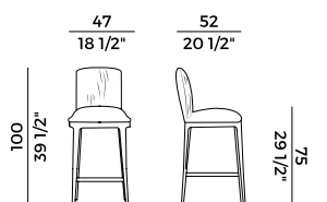
840/A sgabello alto \ barstool
