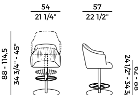
840/AP-GAS sgabello \ stool
