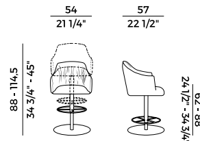
840/AP-GAS sgabello \ stool
