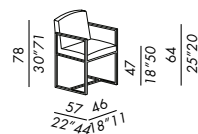
sedia - chair CINQUE
