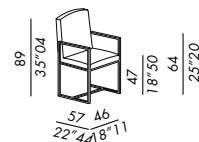
sedia - chair SEI
