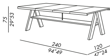
tavolo pranzo / dining table TP-120240
