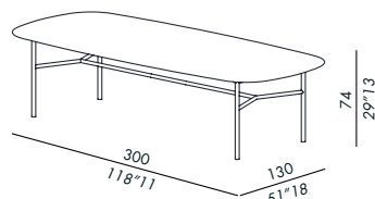
tavolo pranzo - dining table BISCUIT 130300-TP
