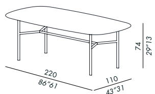
tavolo pranzo - dining table BISCUIT 110220-TP
