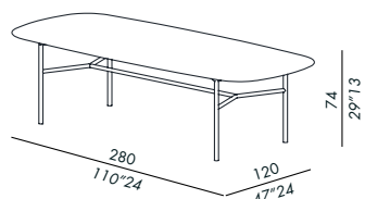
tavolo pranzo - dining table BISCUIT 120280-TP
