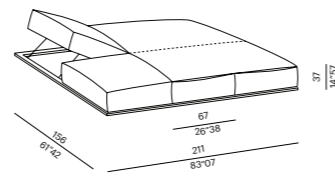
appoggiatesta - bolster
