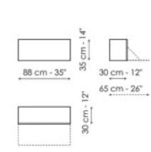
Box Width: 88cm Depth: 30cm Height: 35cm
