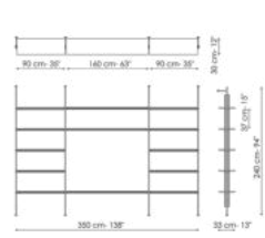
Wall fixing tv-stand module Width: 350cm Depth: 33cm Height: 240cm
