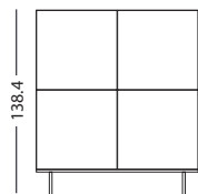
138.4 120.4 Komoda wysoka K2D4 wersja 2 głębokość 48
